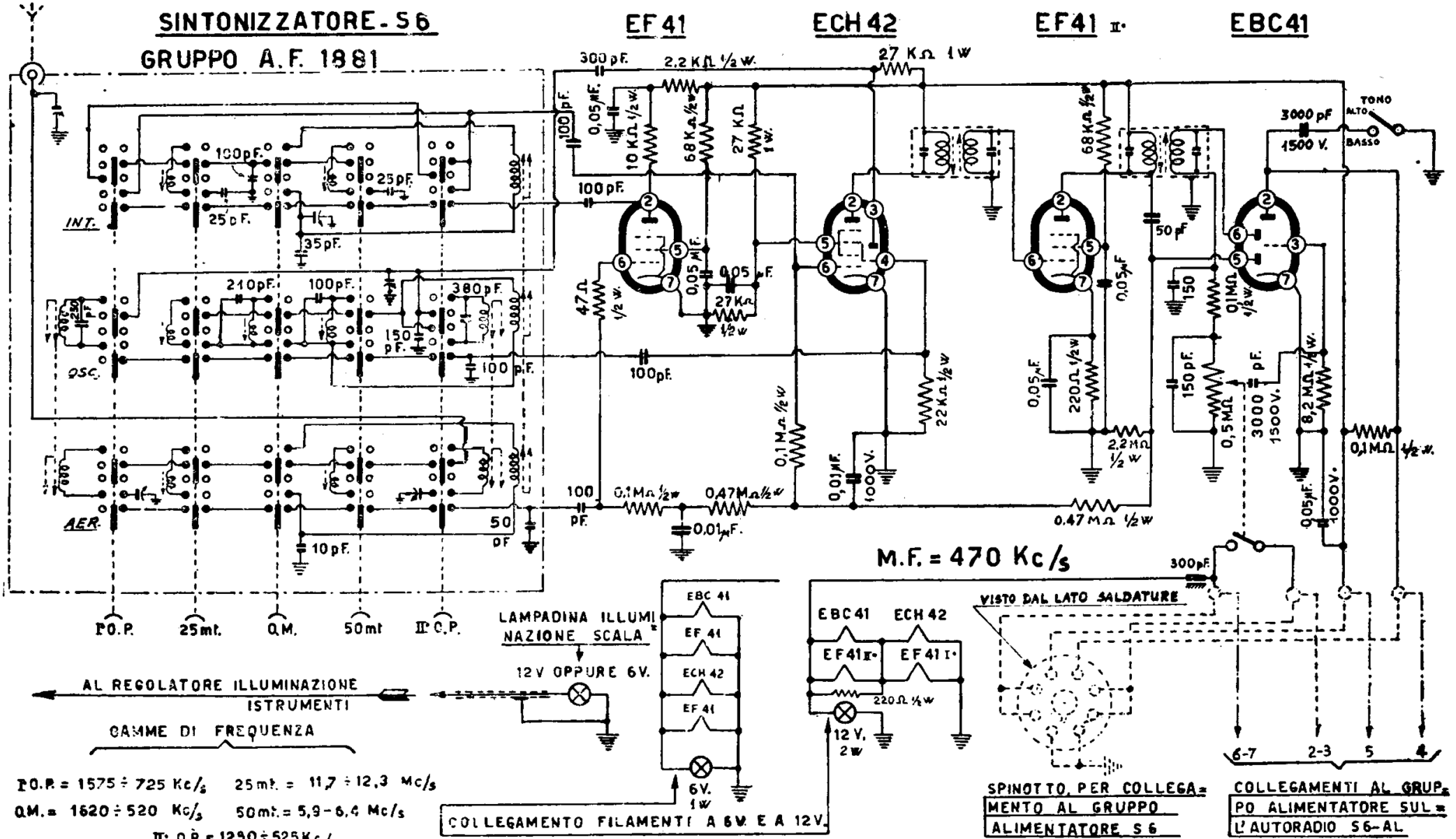
GALLO-CONDOR - Mod. S6. Una gamma onde medie e due ad onde corte. Commutazione di gamma a pulsanti. Media frequenza 470 kc/s. (V. stadio finale ed alimentatore a pag. 79).
